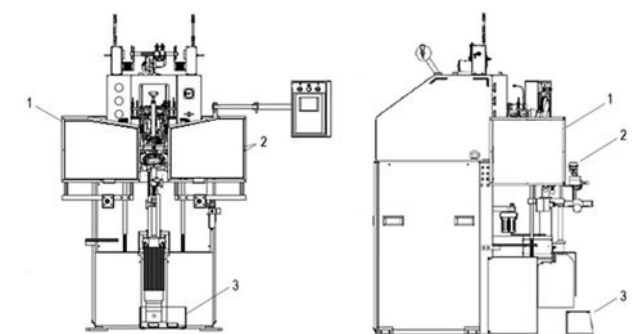
Figura 21: Máquina de alta frequência com mesa móvel manual
