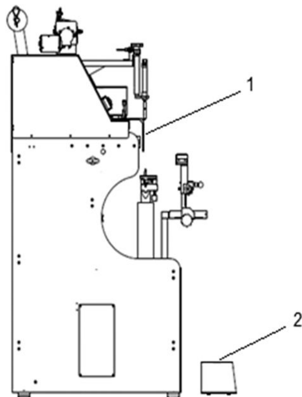
Figura 19: Máquina de montar base de calçados - vista lateral
