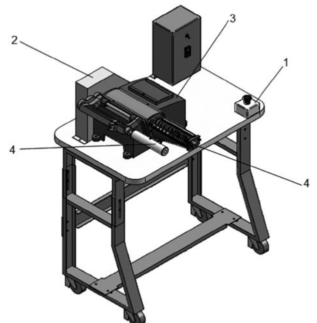
Figura 31: Máquina de passar cola
